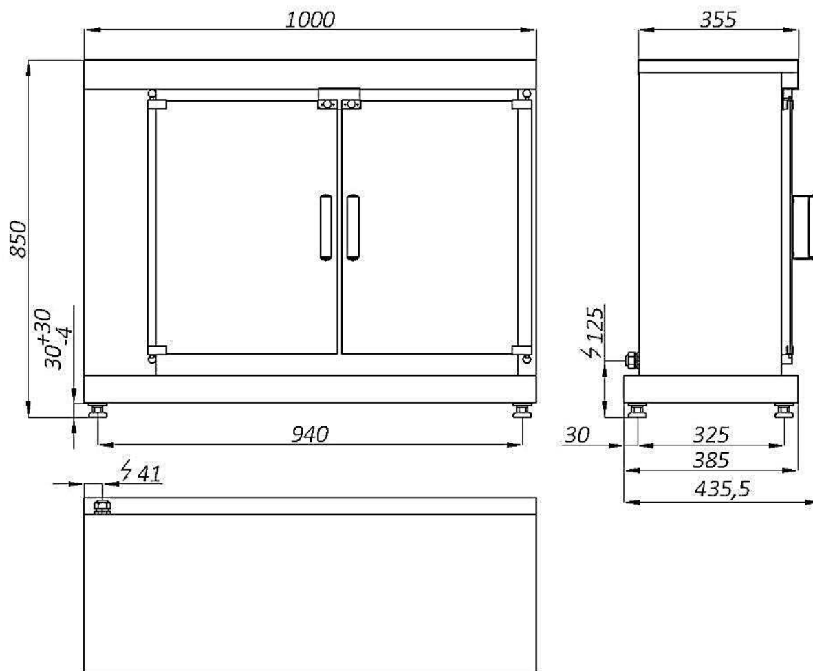
rys 2. Wymiary 000.OE-12
