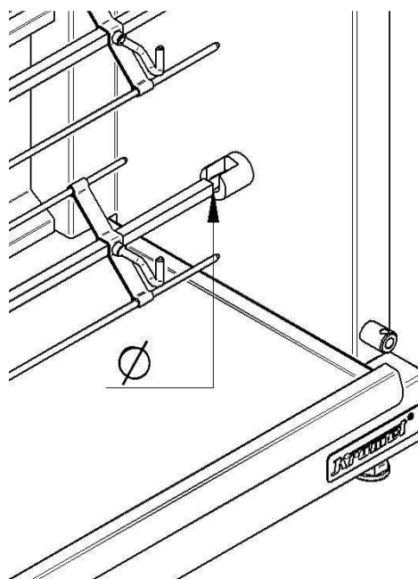
rys 6. Schemat montażu widelca/koszyka strona prawa komory
