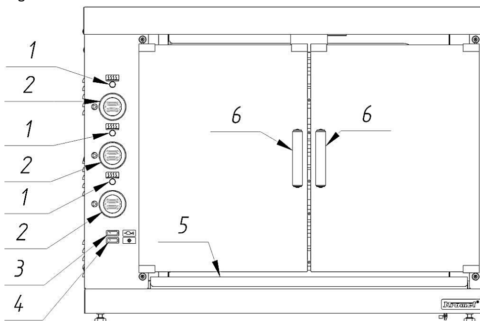
rys 1. Widok ogólny 000.OE-12
