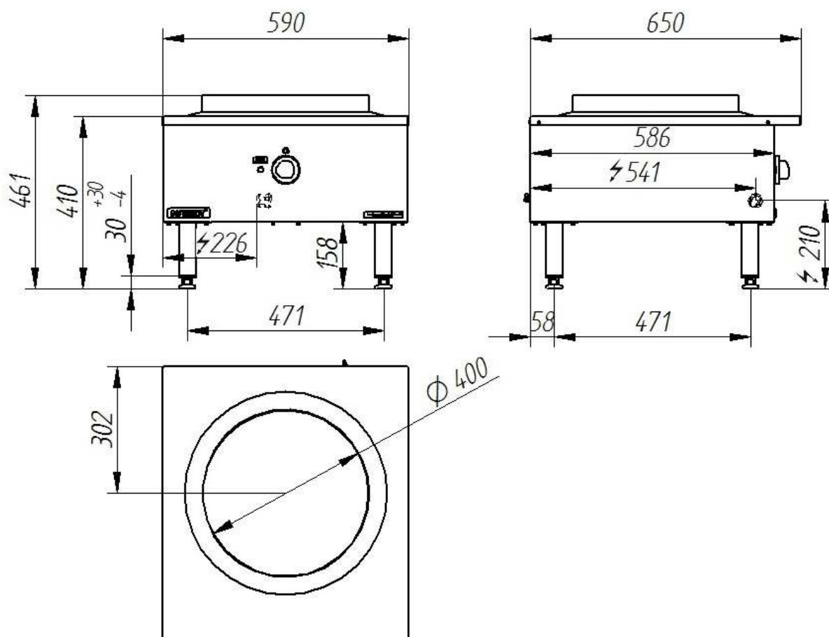
rys 4. Wymiary 000.TE-1F
