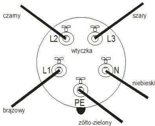
rys 2. Schemat podłączenia przewodu od taboretu do wtyczki
