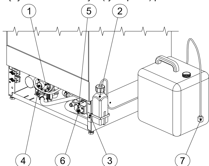
Rys.5 - Podłączenie do zbiorników
