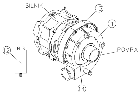
Rys. 19 - Zespół pompy mycia
