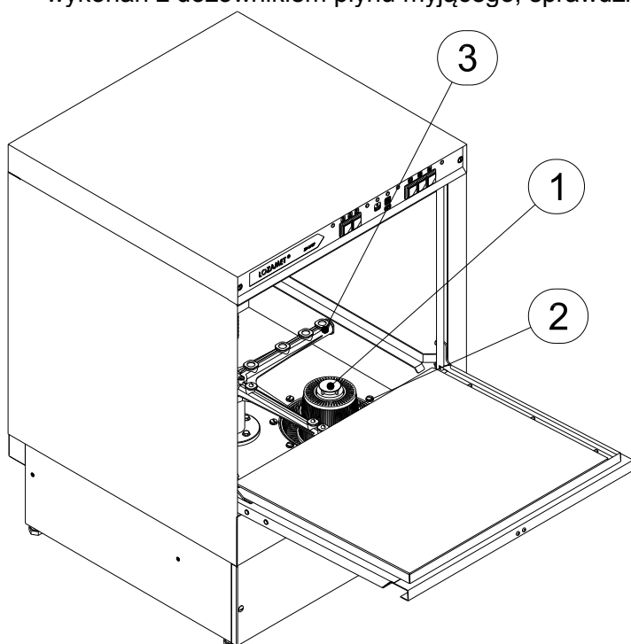
Rys. 6 - Widok komory mycia
