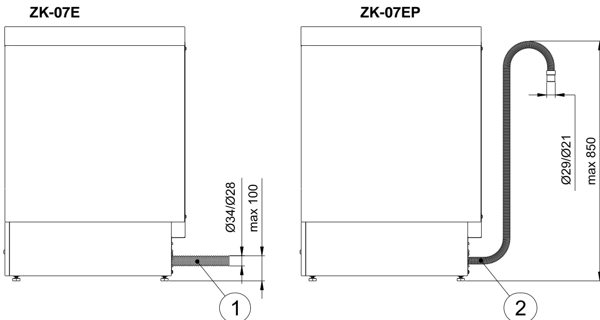
Rys.4 - Wąż spustowy wody
