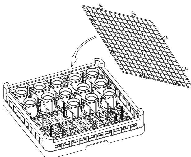
Rys.15 - Kratka PK1 z koszem PV 251
