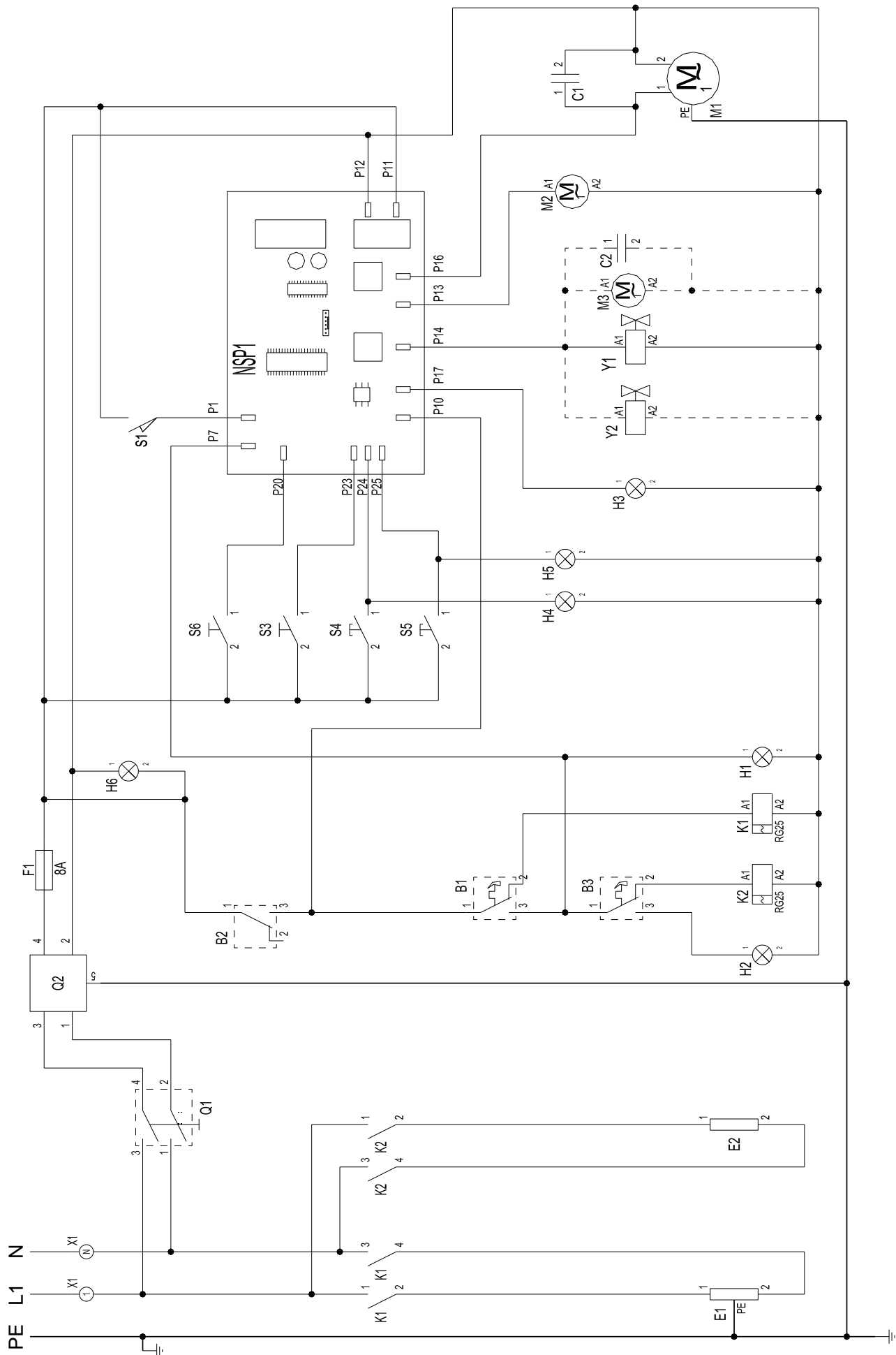
Sch. 4- Schemat instalacji elektrycznej zmywarki ZK.07.4EP
