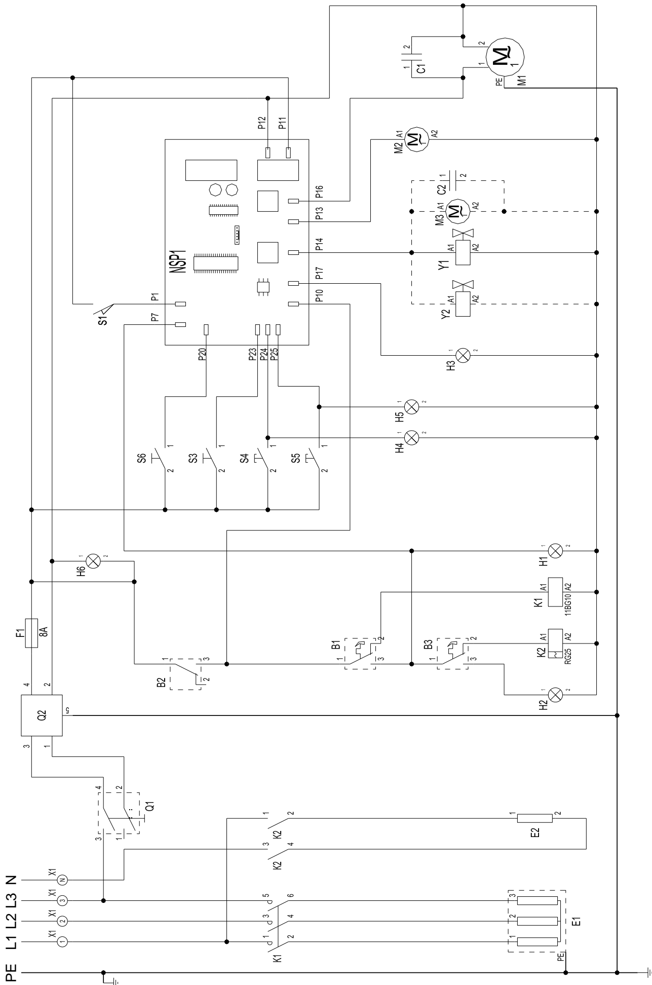
Sch. 6- Schemat instalacji elektrycznej zmywarki ZK.07.5EP i ZK.07.6EP
